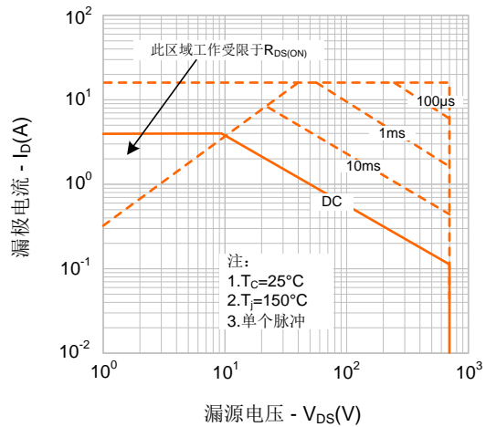
图9-2. 最大安全工作区域(SVF4N70D)
